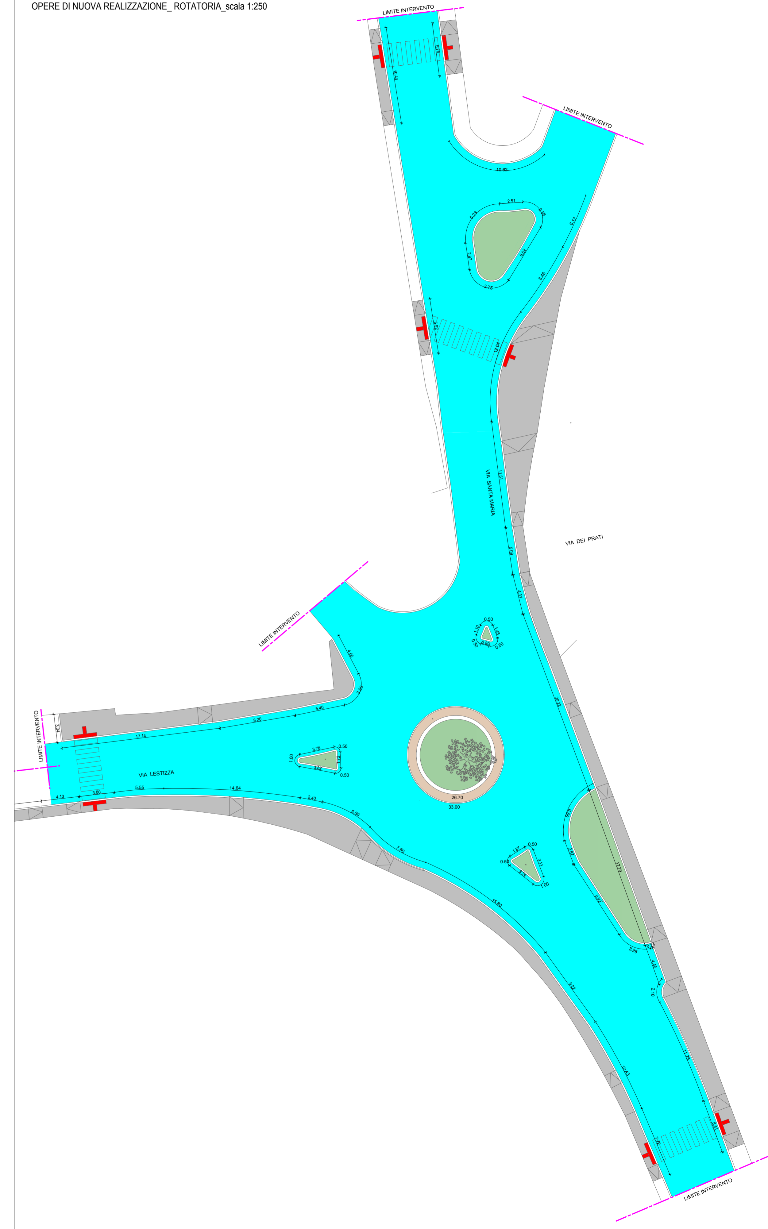
OPERE DI NUOVA REALIZZAZIONE_ ROTATORIA_scala 1:250
