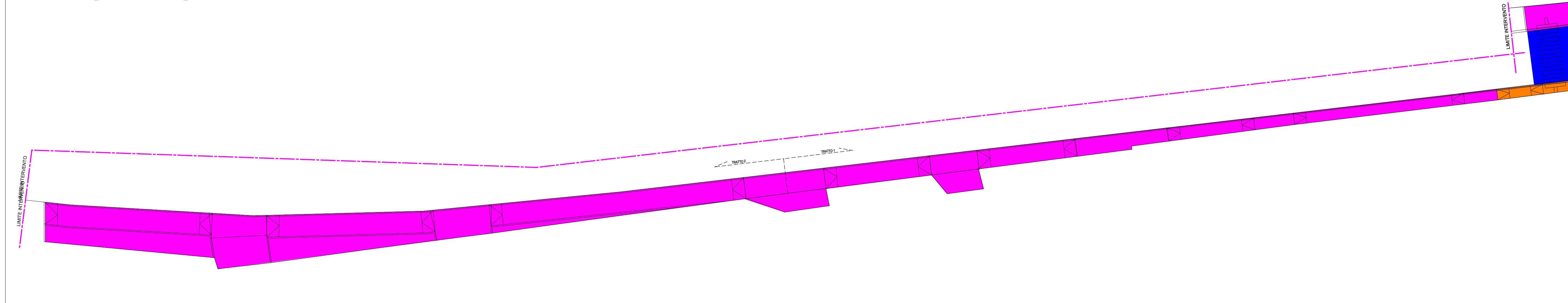
OPERE DA DEMOLIRE_ PISTA CICLOPEDONALE_ scala 1:250
